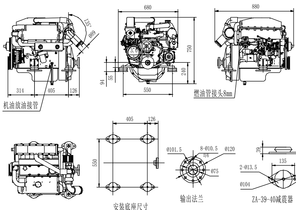
SY144C 外形安装图
